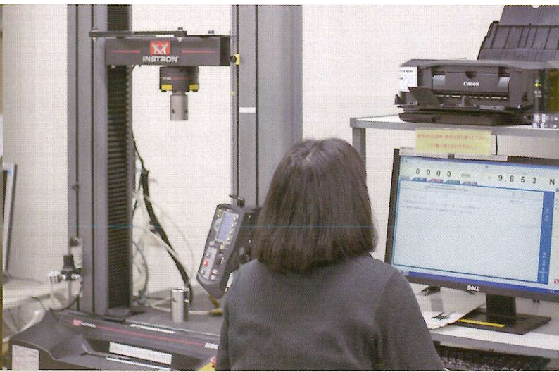
万能材料試験機10kN
