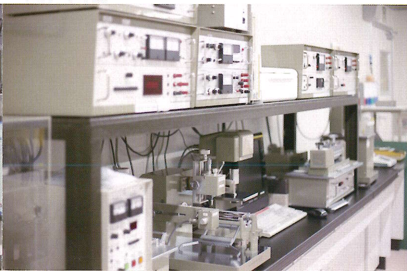
風合い試験機
